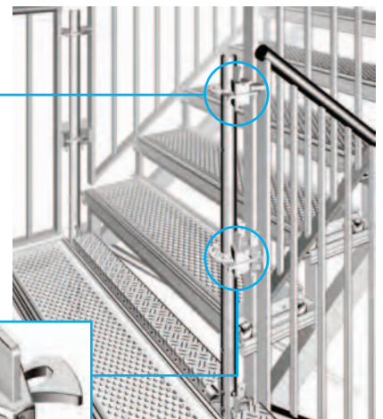
Fijación para barandilla interior Ref. n.º 2636.000
