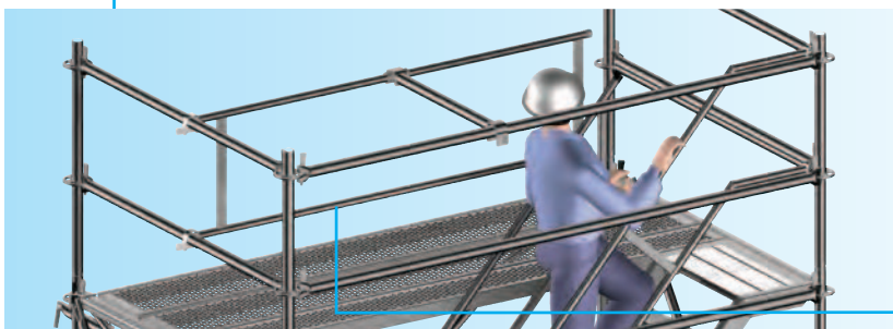
Barandilla interior de terminación de escalera Ref. n.º 0718.592
